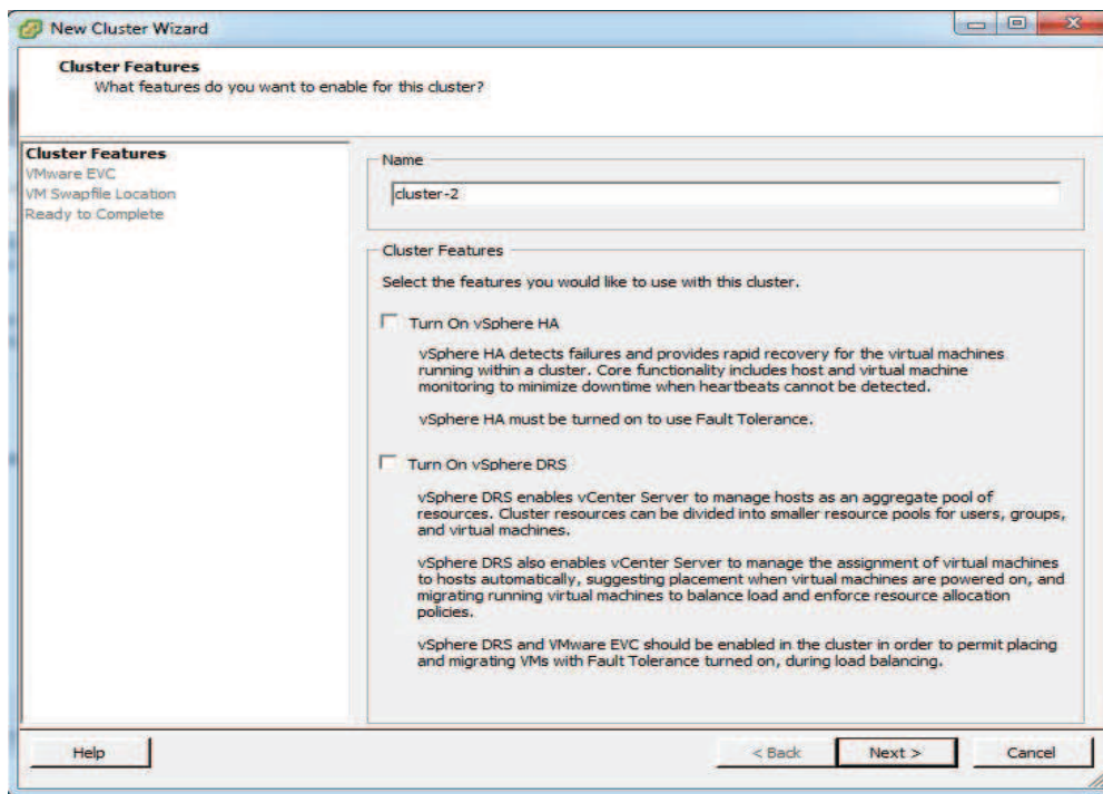
شکل 3-6. ساخت کلاستر
