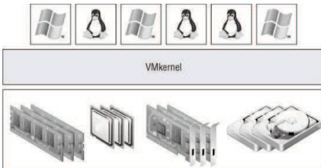
شکل 1-3 . ساختار ESXi
